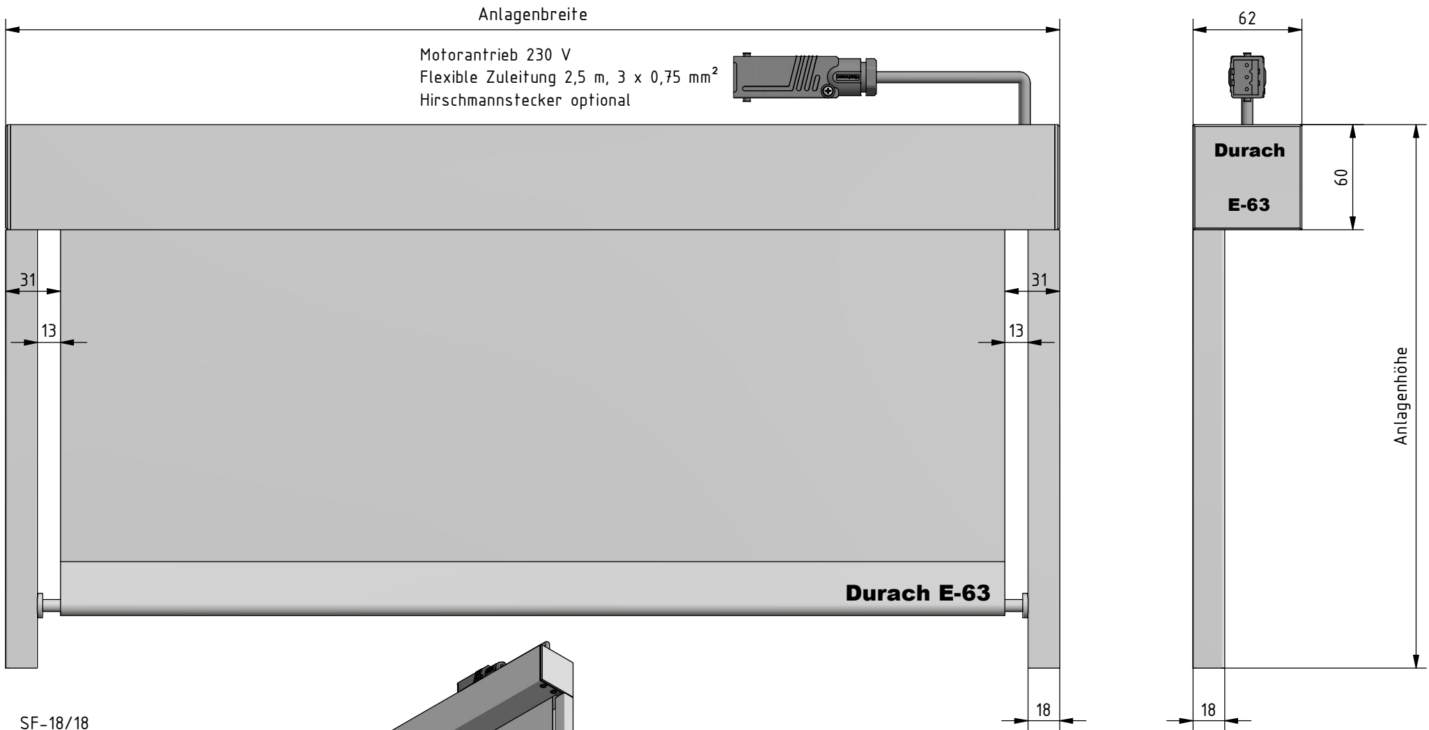
SF-18/18 Maßstab (1 : 1)
